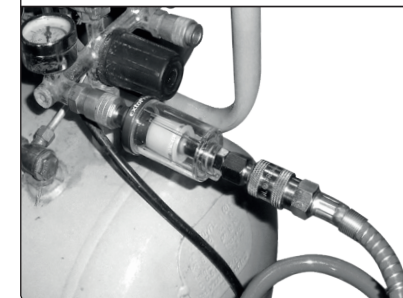
Obr. 6, pripojenie filtra (odlučovača) Extol® Craft 8865101
