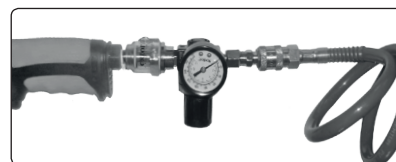
5. ábra. Bekötési vázlat
